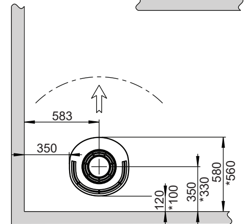
Brännbar vägg
