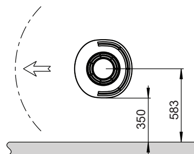
Avstånd till brännbar vägg med vridbar pelare:
