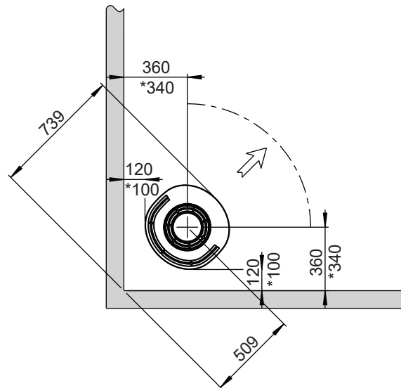
Min. avstånd til brännbar vägg
