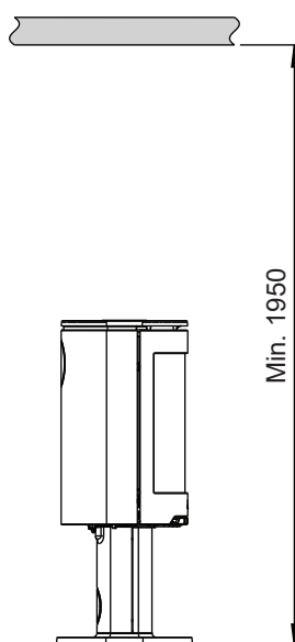
Brännbart tak
