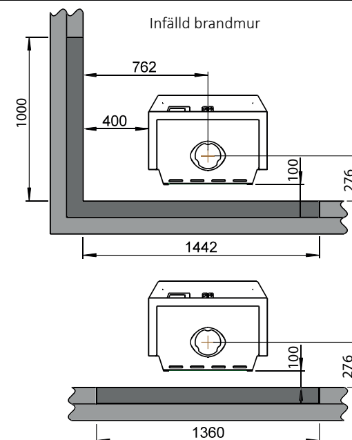
Infälld brandmur
