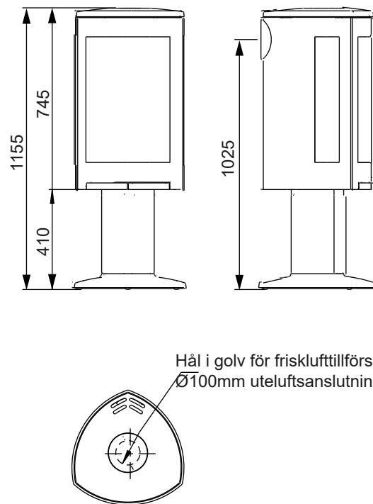
Jøtul F 373 Advance
