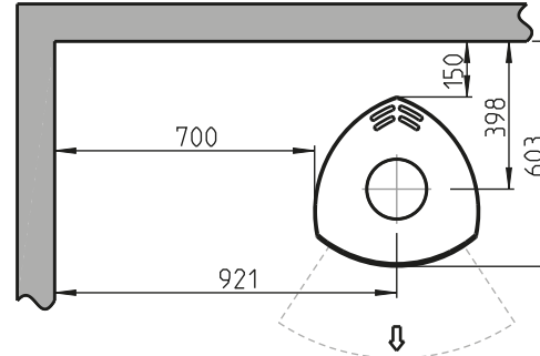
Min. avstånd till brännbar vägg
